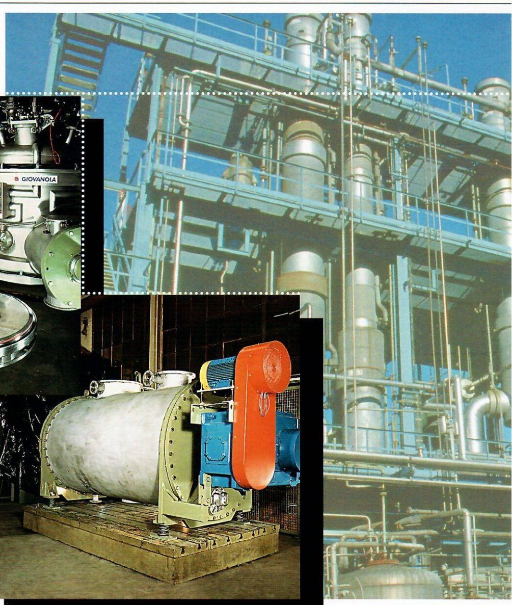
Sécheur à palettes Paddle dryer Schaufeltrockner
