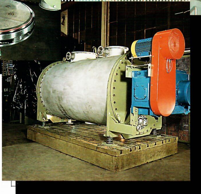
Sécheur à palettes Paddle dryer Schaufeltrockner
