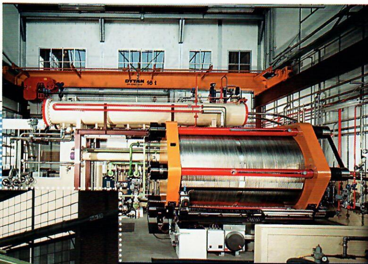
Electrolyseur atmosphérique Atmospheric electrolyser Atmosphärischer Elektrolyseur
